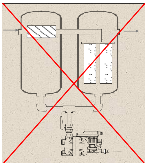
圖12 排水器安裝不應二組共用
