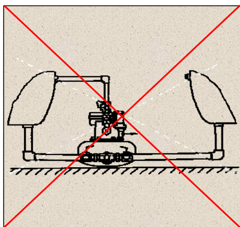
圖13 排水器安裝不應二組共用且大氣量需獨立回氣管
