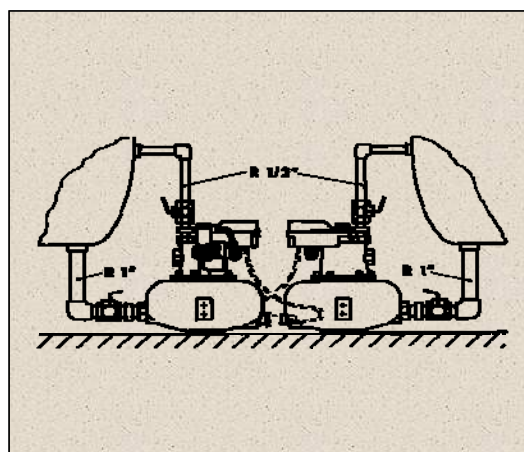
圖13 排水器安裝不應二組共用且大氣量需獨立回氣管
