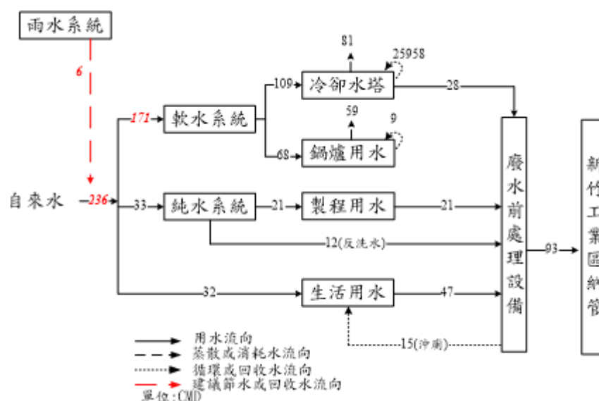
圖 39 案例 A 廠用水平衡圖（方案實施後）
