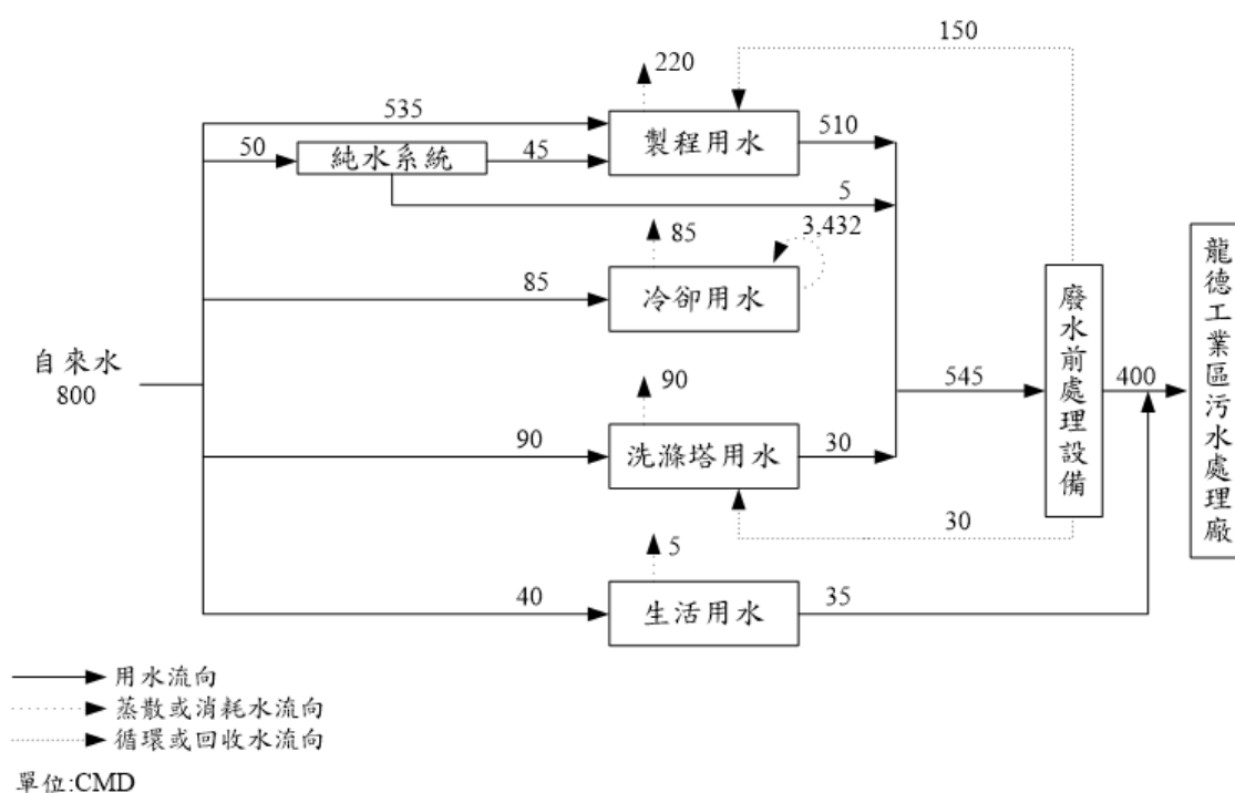
■ 圖 42 案例 A 廠用水平衡圖（方案實施前）
