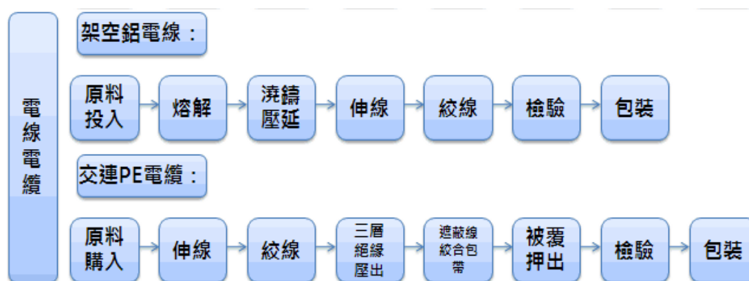
圖 4 電線電纜製造流程圖
