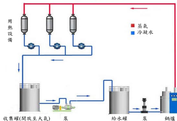
■ 圖 26 開放式冷凝水回收系統原理示意圖
