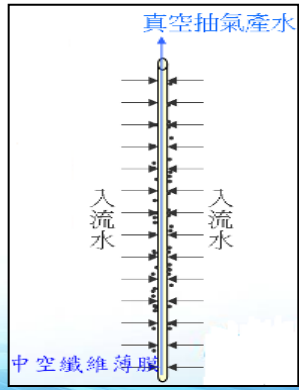
MBR膜產水動作
